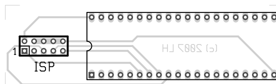
Fig. 6: Adaptateur 40 broches face composants
