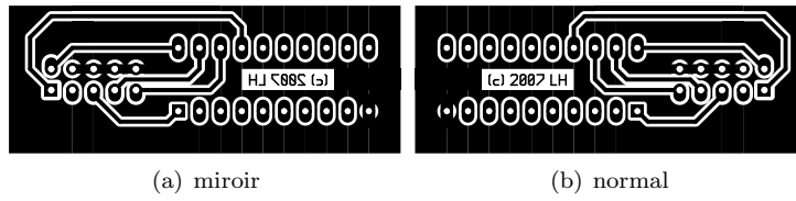
Fig. 1: Adaptateur 20 broches face soudure
