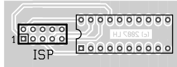
Fig. 2: Adaptateur 20 broches face composants
