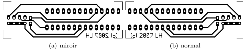
Fig. 3: Adaptateur 28 broches face soudure
