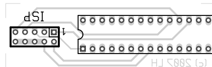
Fig. 4: Adaptateur 28 broches face composants
