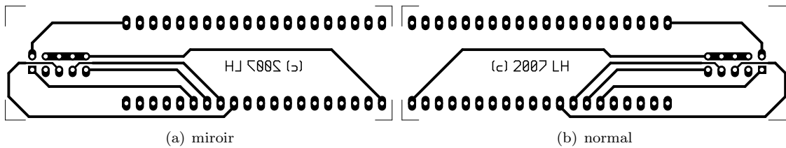
Fig. 5: Adaptateur 40 broches face soudure
